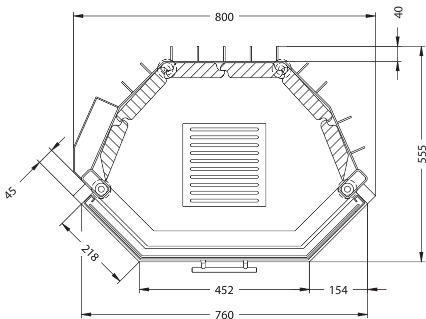
Horizontalschnitt M~1:10
