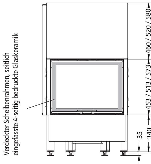
Vorderansicht M~1:20
