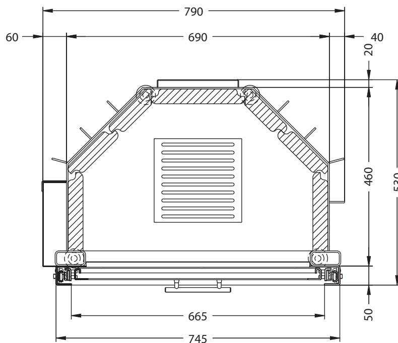
Horizontalschnitt M~1:10
