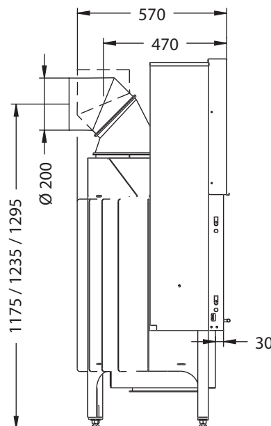
Seitenansicht M~1:20
