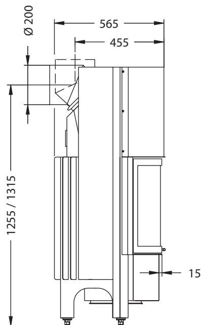
Seitenansicht M~1:20
