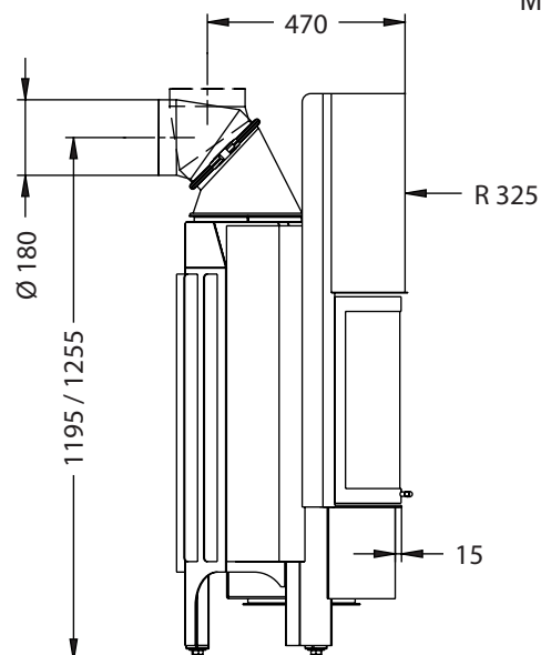
Seitenansicht M~1:20
