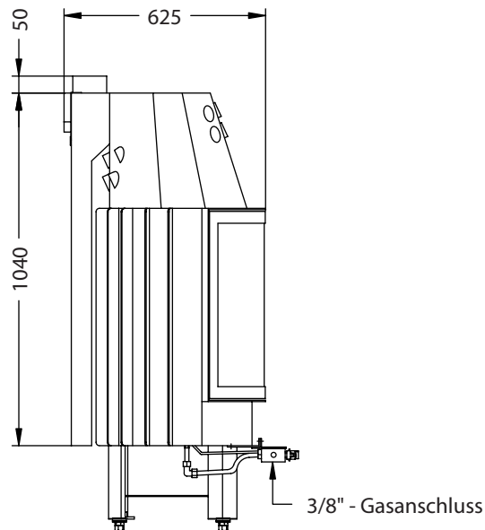
Seitenansicht M~1:20
