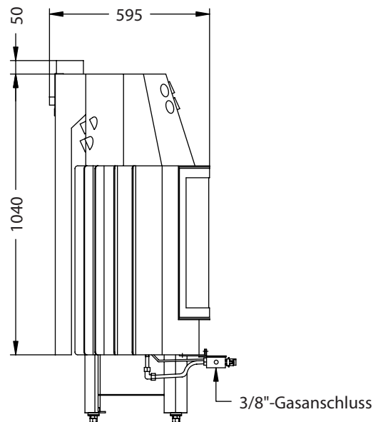
Seitenansicht M~1:20
