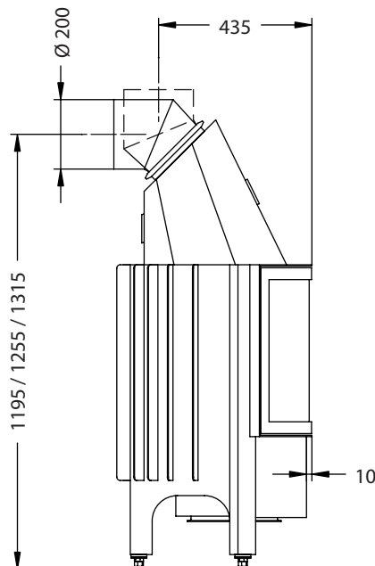
Seitenansicht M~1:20
