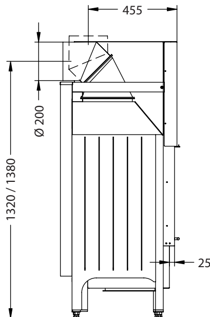
Seitenansicht M~1:20
