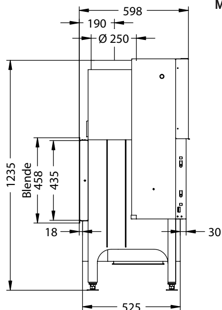
Seitenansicht M~1:20
