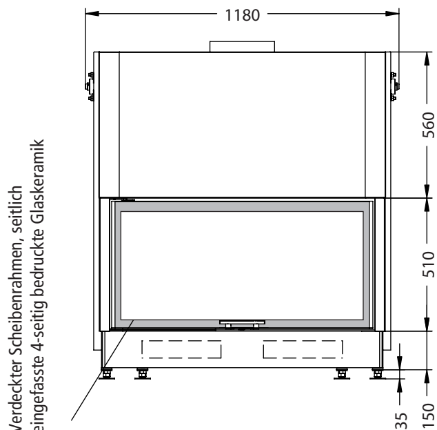
Vorderansicht M~1:20
