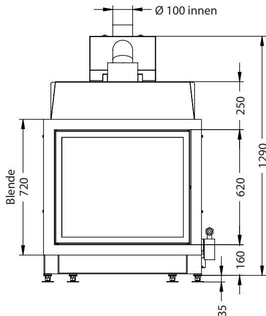
Vorderansicht M~1:20
