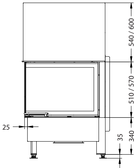
Vorderansicht M~1:20
