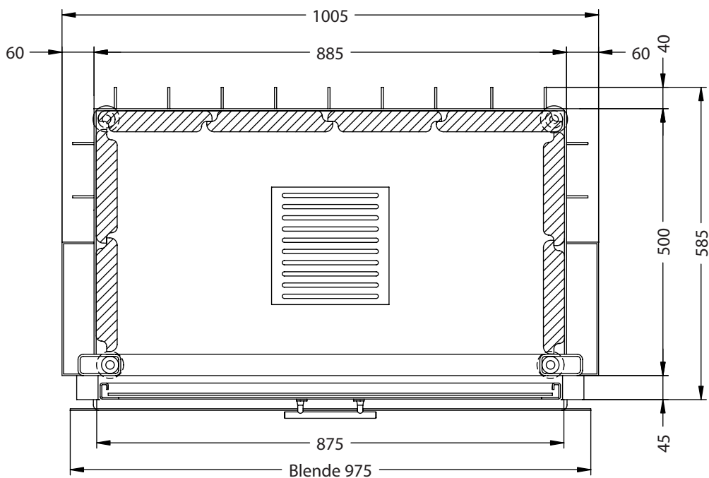
Horizontalschnitt M~1:10
