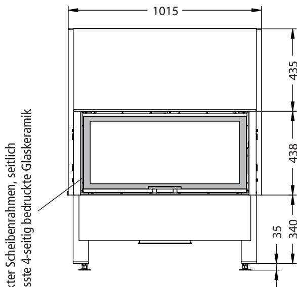
Vorderansicht M~1:20
