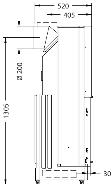
Seitenansicht M~1:20
