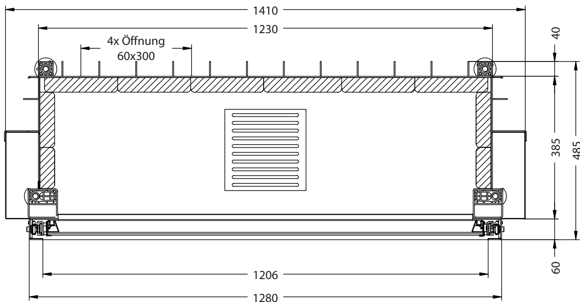
Horizontalschnitt M~1:10
