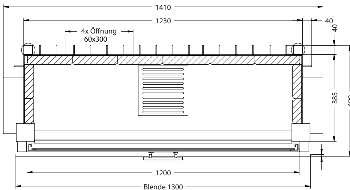
Horizontalschnitt M~1:10
