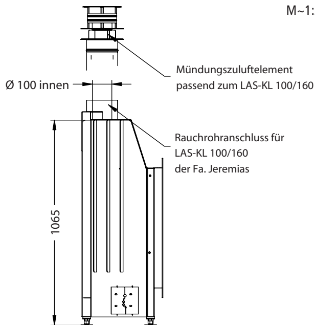
Seitenansicht M~1:20
