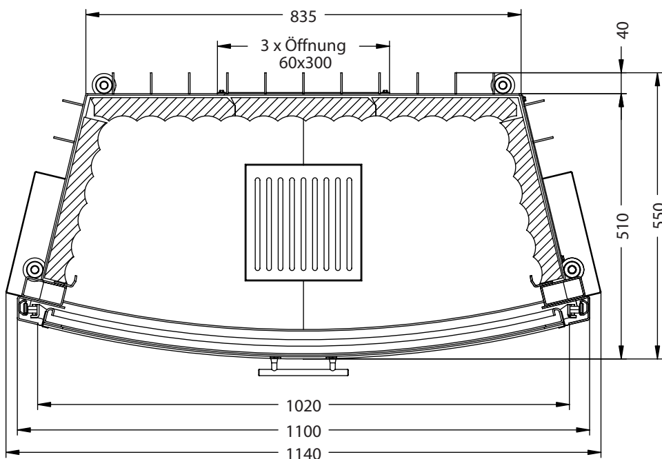
Horizontalschnitt M~1:10
