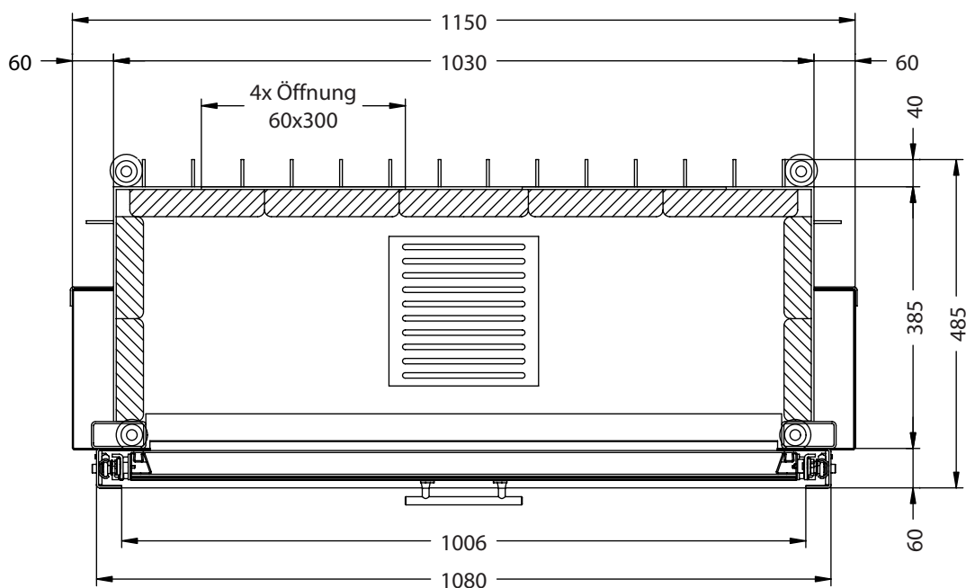
Horizontalschnitt M~1:10
