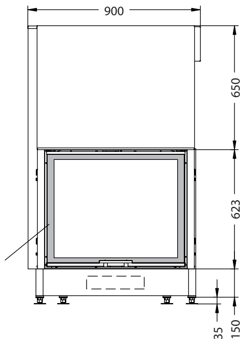
Vorderansicht M~1:20
