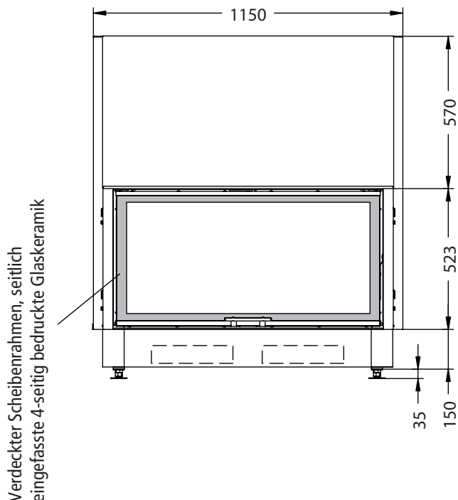
Vorderansicht M~1:20
