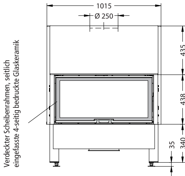
Vorderansicht M~1:20
