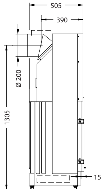
Seitenansicht M~1:20
