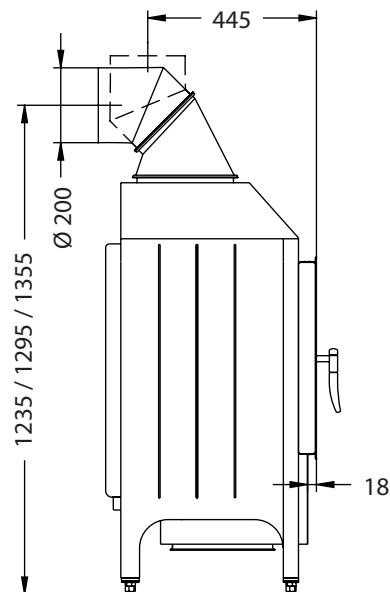
Seitenansicht M~1:20
