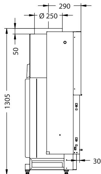
Seitenansicht M~1:20
