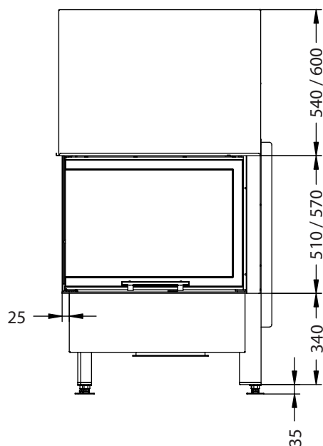
Vorderansicht M~1:20
