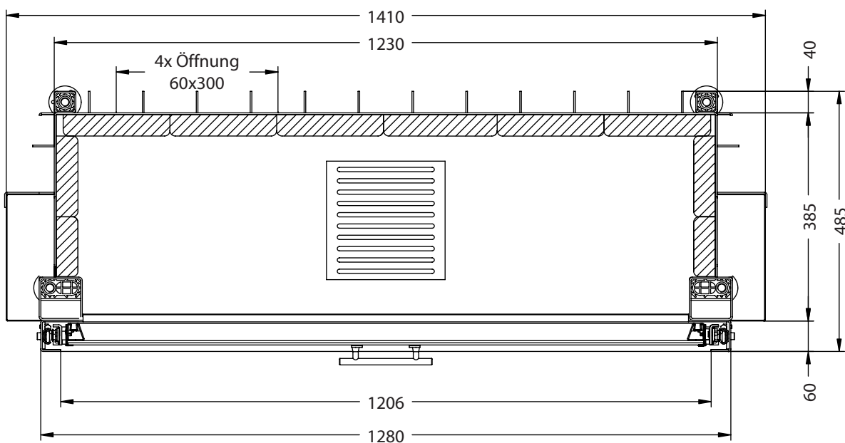
Horizontalschnitt M~1:10
