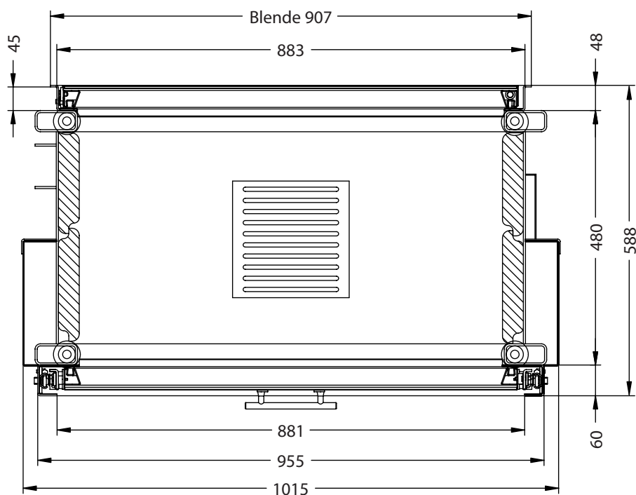
Horizontalschnitt M~1:10
