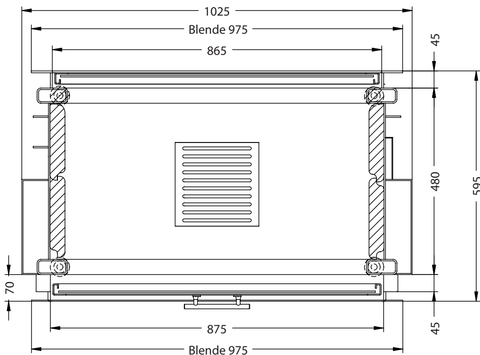
Horizontalschnitt M~1:10
