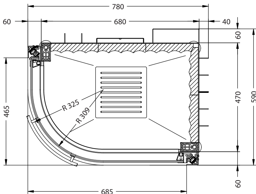
Horizontalschnitt M~1:10
