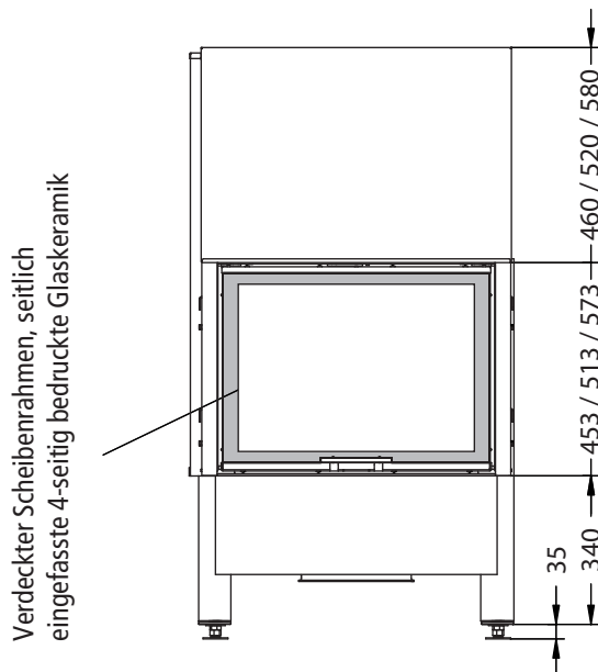
Vorderansicht M~1:20
