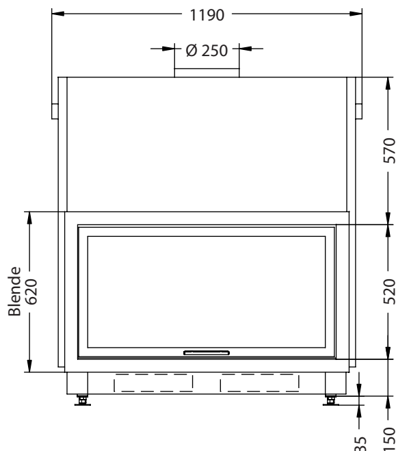
Vorderansicht M~1:20
