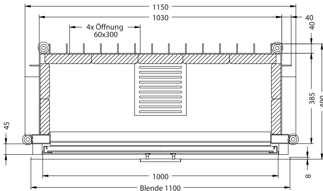
Horizontalschnitt M~1:10
