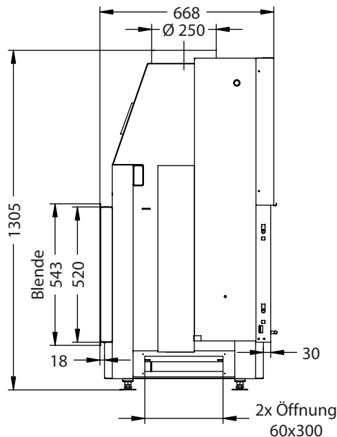
Seitenansicht M~1:20
