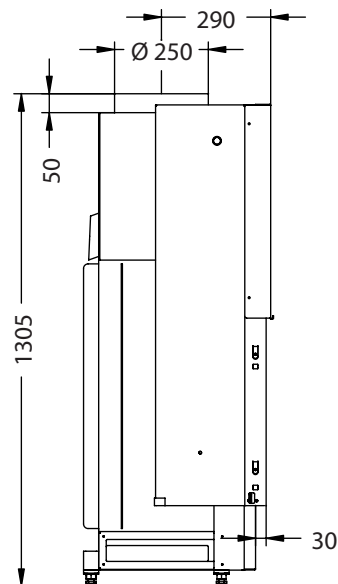
Seitenansicht M~1:20
