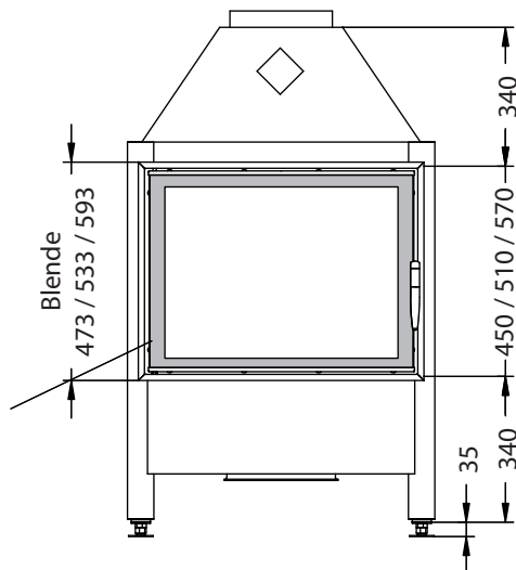
Vorderansicht M~1:20
