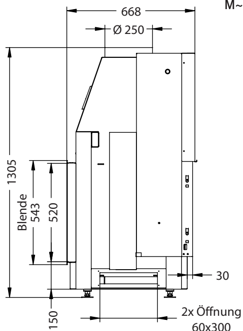
Seitenansicht M~1:20
