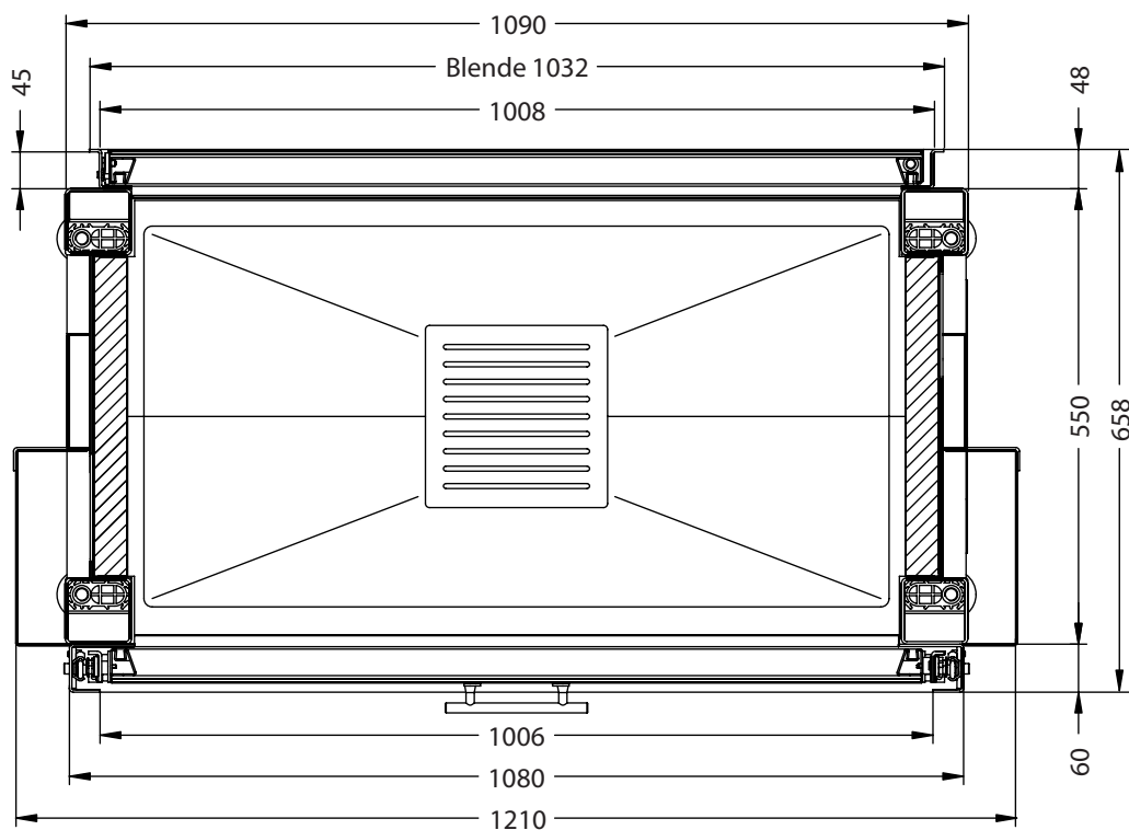
Horizontalschnitt M~1:10
