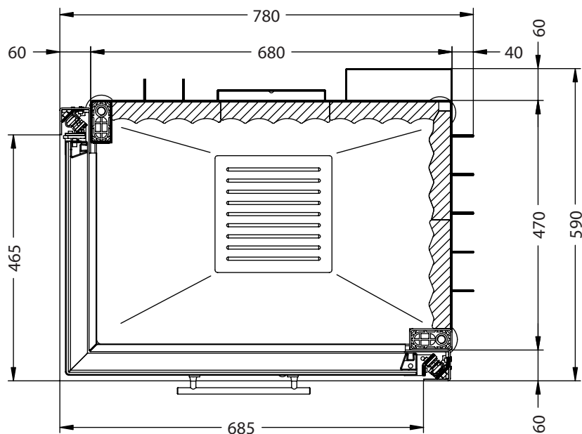
Horizontalschnitt M~1:10
