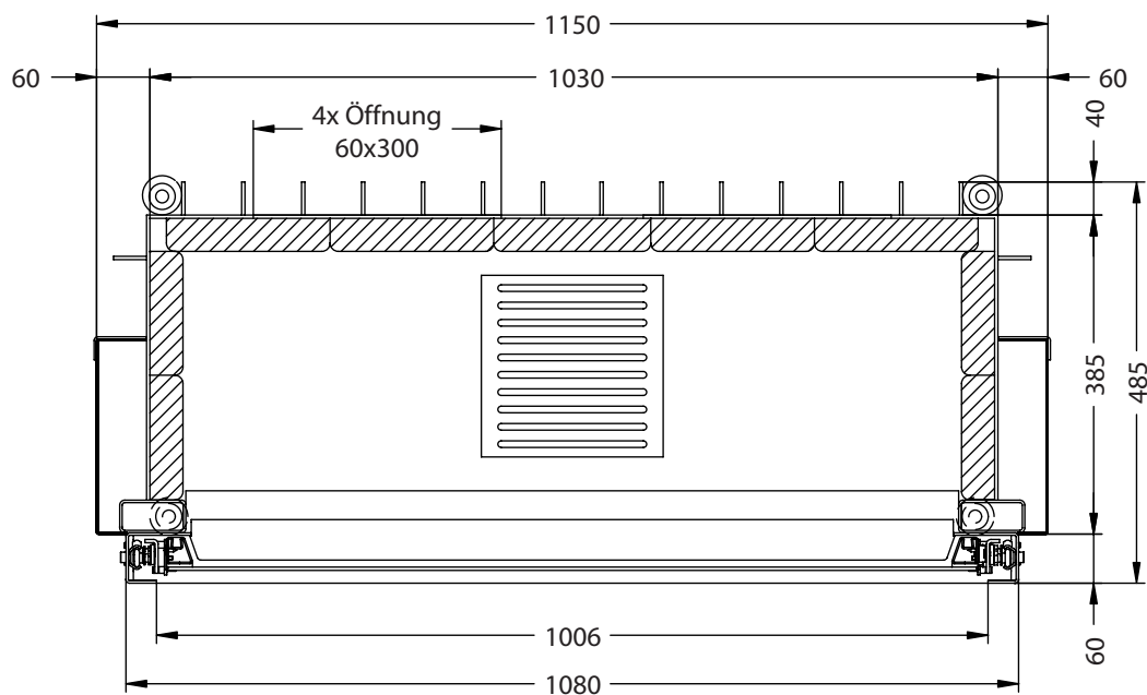
Horizontalschnitt M~1:10
