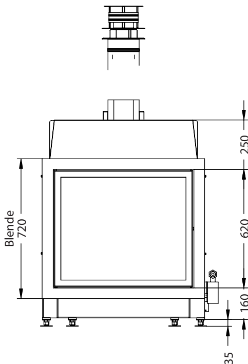
Vorderansicht M~1:20
