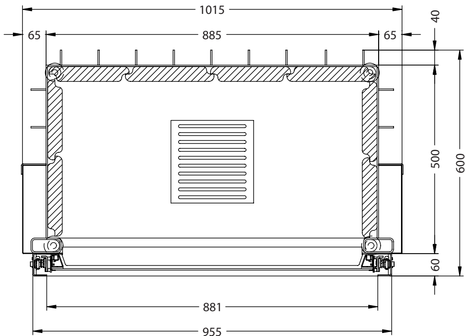
Horizontalschnitt M~1:10
