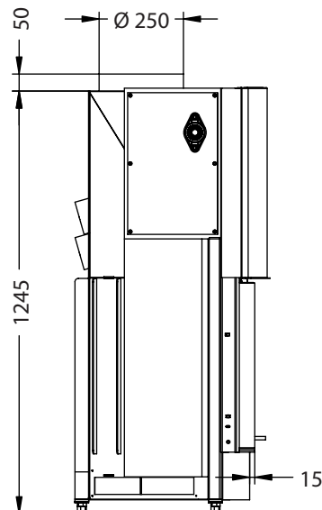
Seitenansicht M~1:20
