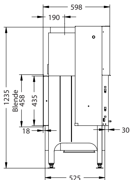
Seitenansicht M~1:20
