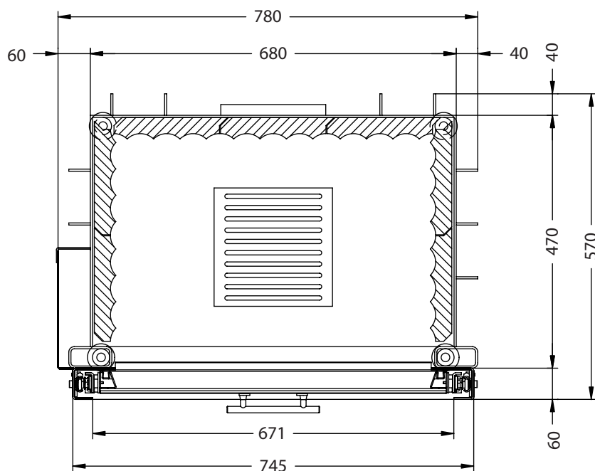
Horizontalschnitt M~1:10
