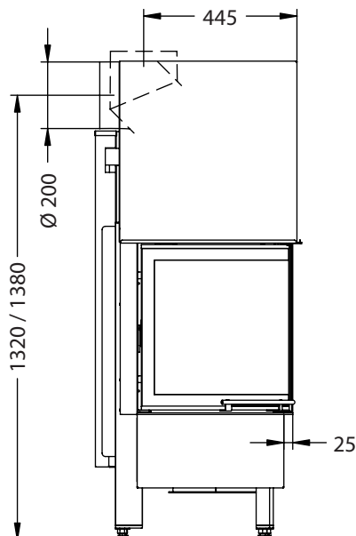
Seitenansicht M~1:20
