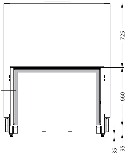
Vorderansicht M~1:20
