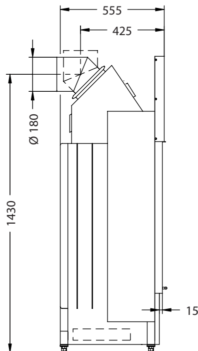
Seitenansicht M~1:20
