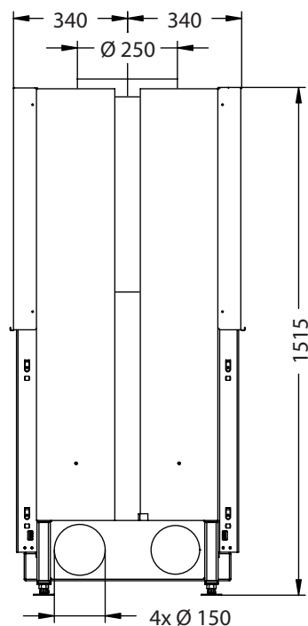
Seitenansicht M~1:20
