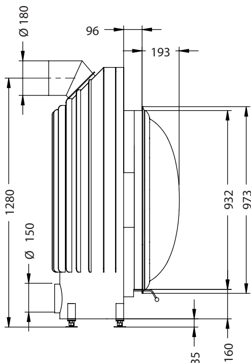
Seitenansicht M~1:20
